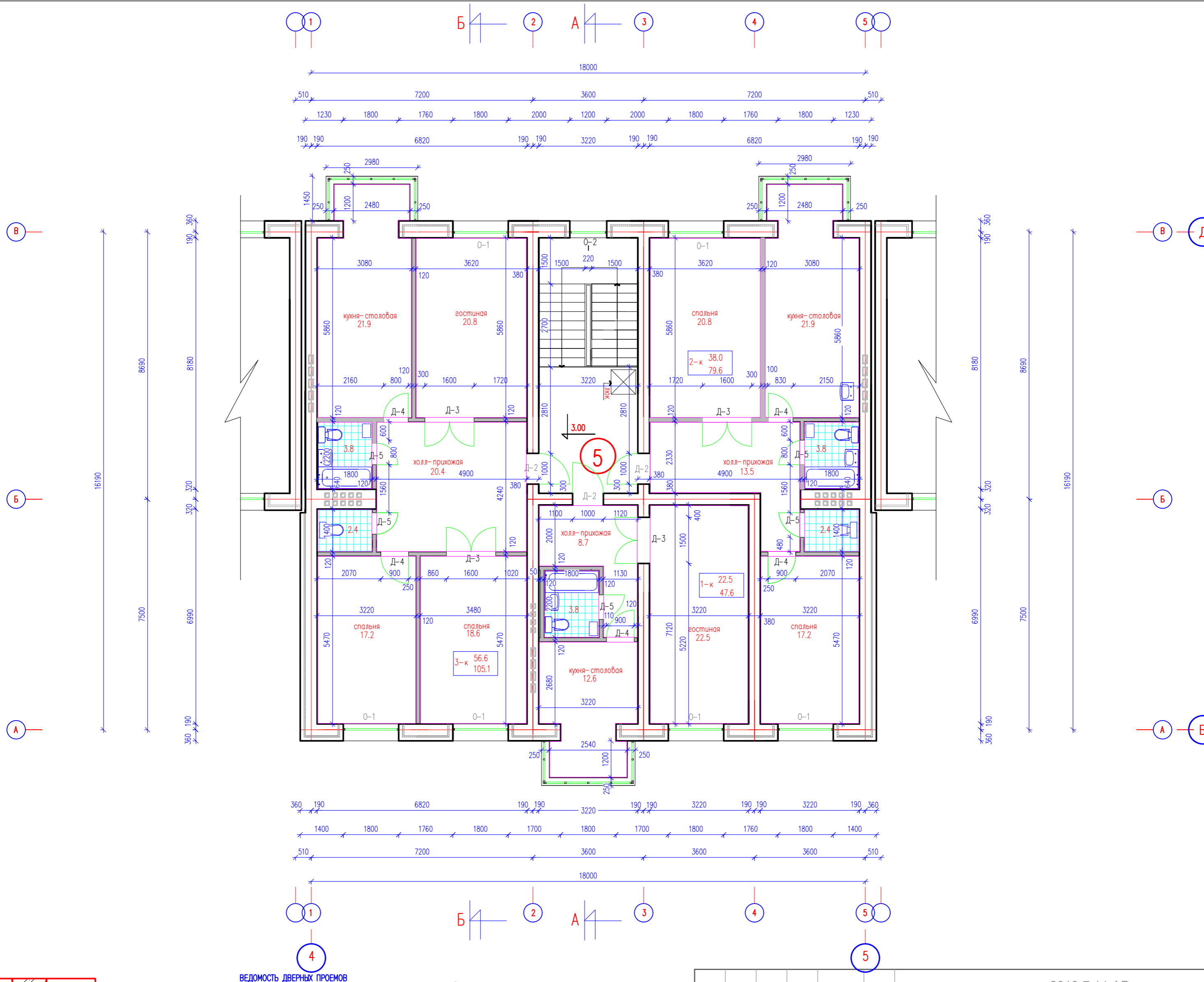
2-этаж
