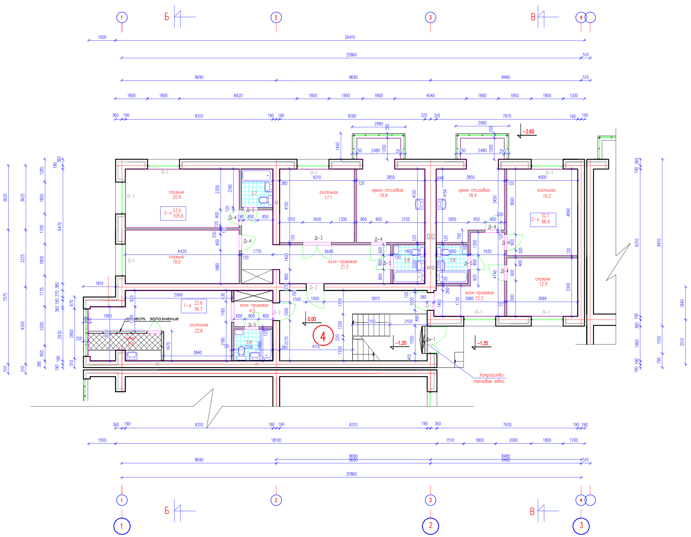
ВЕДОМОСТЬ ДВЕРНЫХ ПРОЕМОВ
