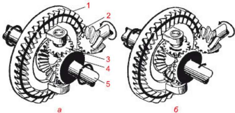
Рис. 4.9. Схема устройства и работы дифференциала:
