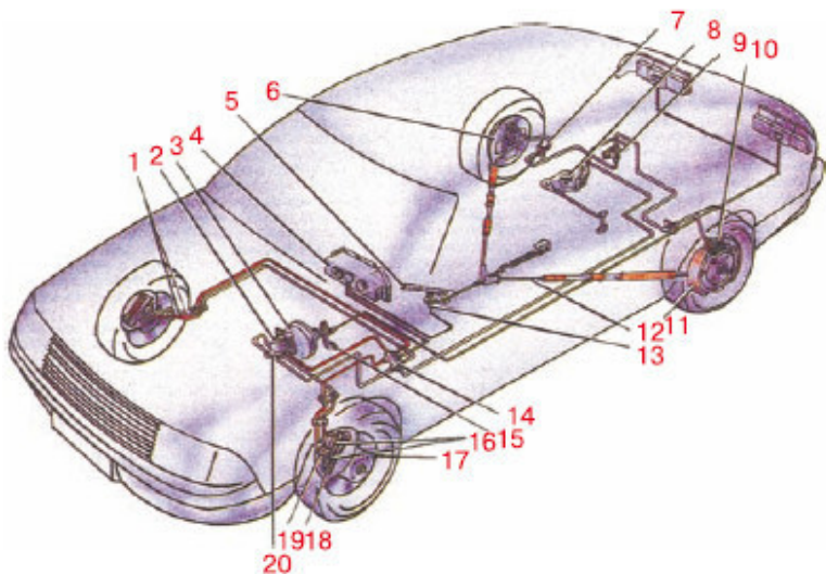
Рис. 6.1. Тормозная система:
