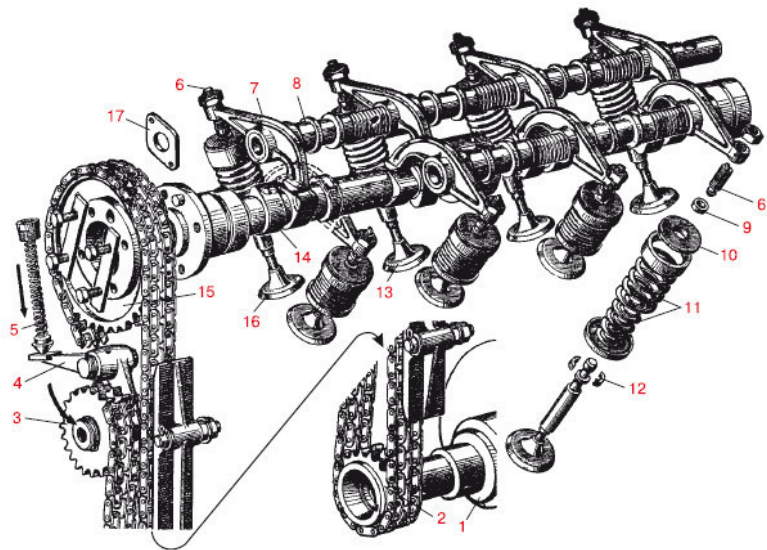
Рис. 2.11. Газораспределительный механизм:
