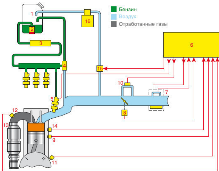
Рис. 2.18. Инжекторная система:
