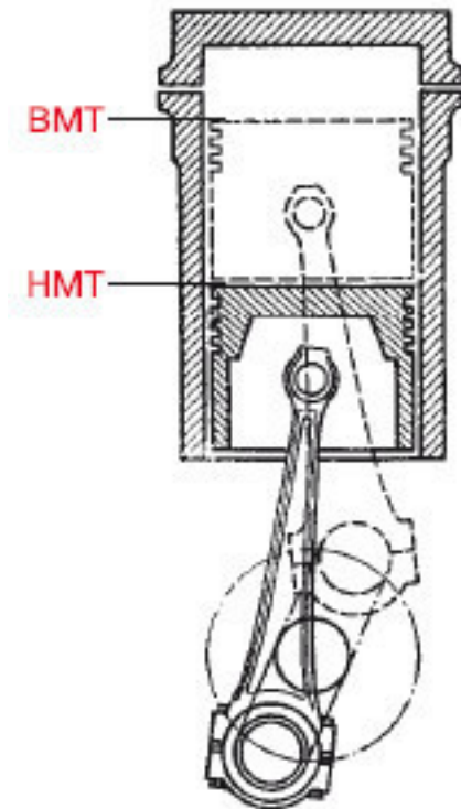
Рис. 2.3. Поршень
