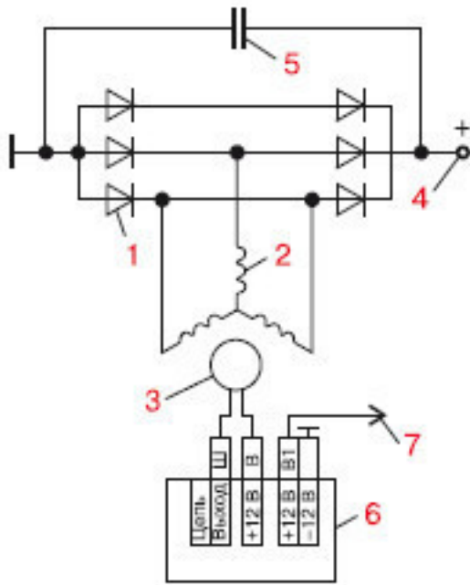
Рис. 3.3. Принципиальная электрическая схема генератора:
