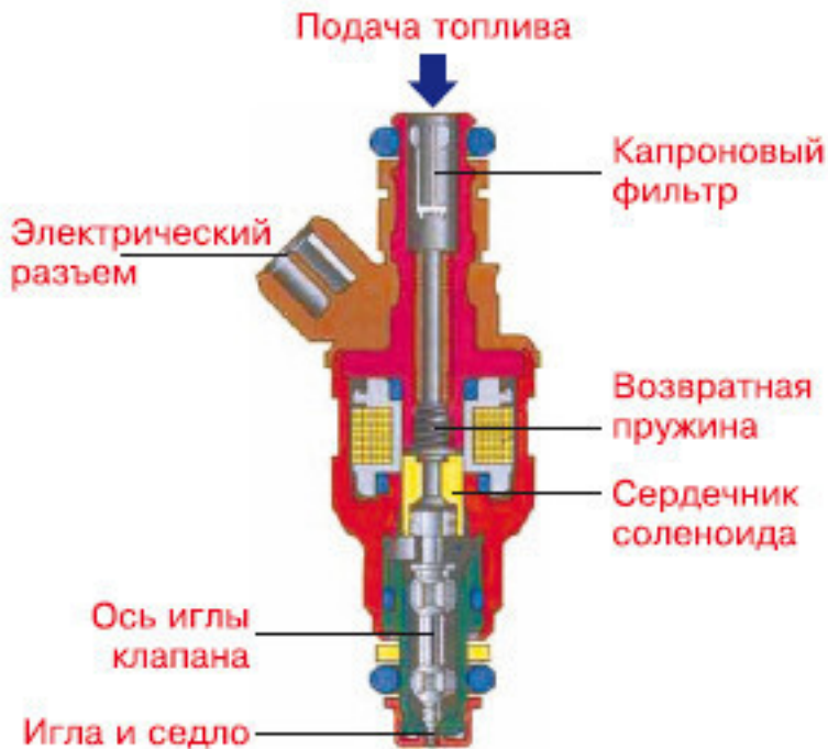
Рис. 2.16. Электромагнитная форсунка
