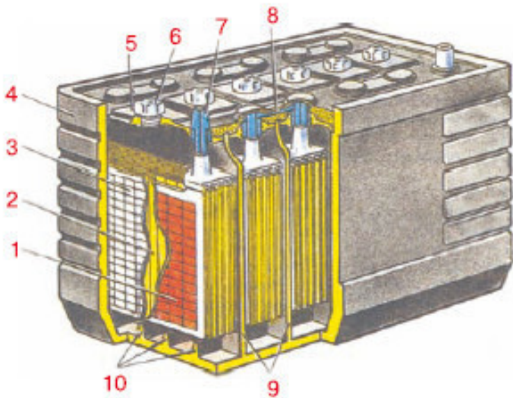
Рис. 3.1. Аккумуляторная батарея:
