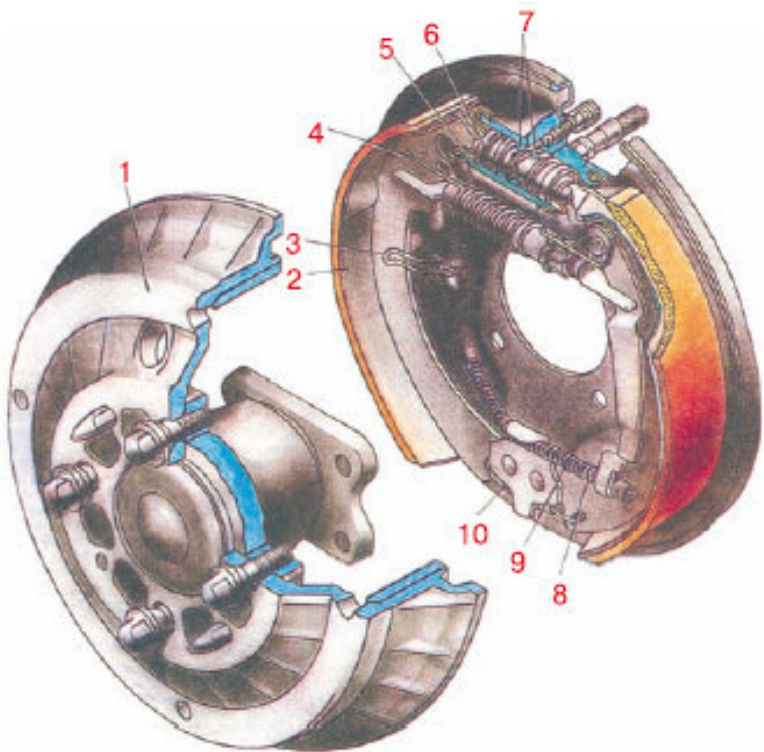
Рис. 6.4. Барабанный тормозной механизм:
