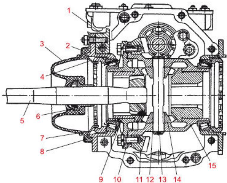
Рис. 4.8. Главная передача и дифференциал заднеприводного автомобиля:
