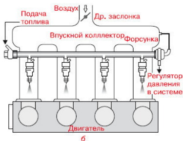
Рис. 2.17. Системы впрыска: а – одноточечная; б – многоточечная
