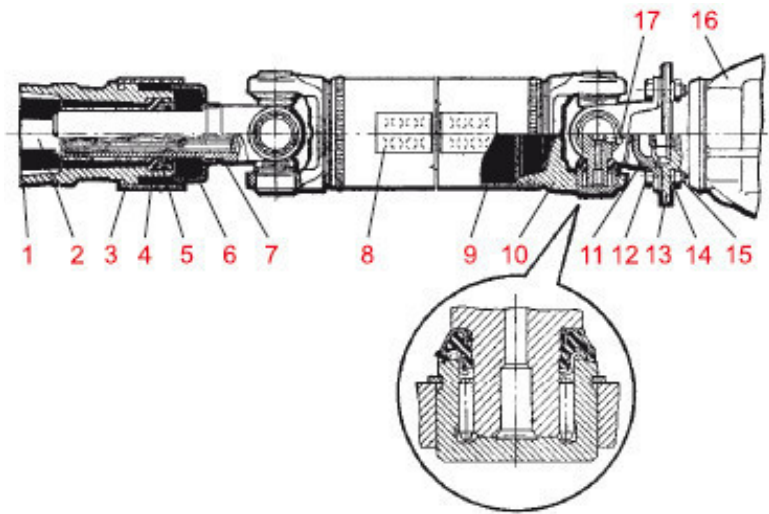
Рис. 4.7. Карданная передача:
