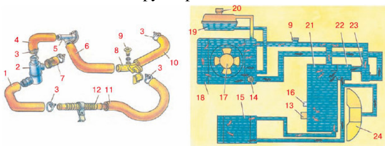
Рис. 2.21. Система охлаждения двигателя:
