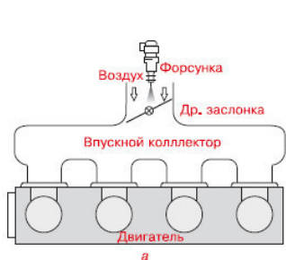
Рис. 2.17. Системы впрыска: а – одноточечная; б – многоточечная
