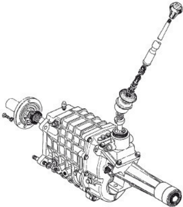
Рис. 4.4. Коробка переключения передач с рычагом
