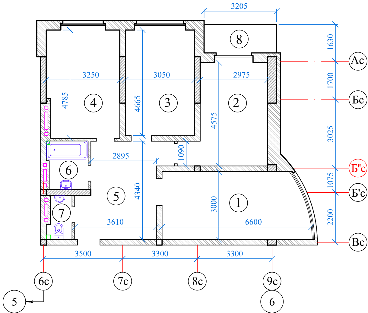
Экспликация помещений
