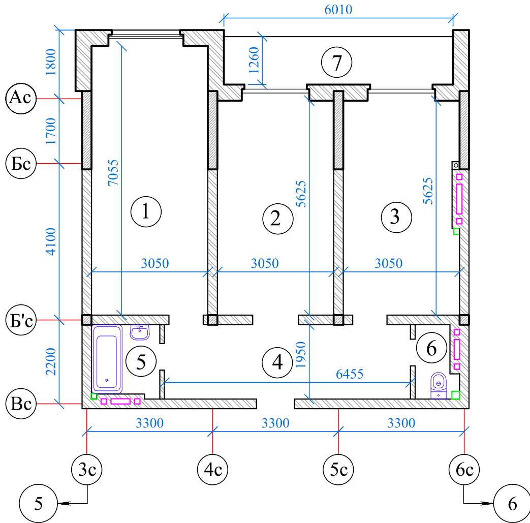
Экспликация помещений
