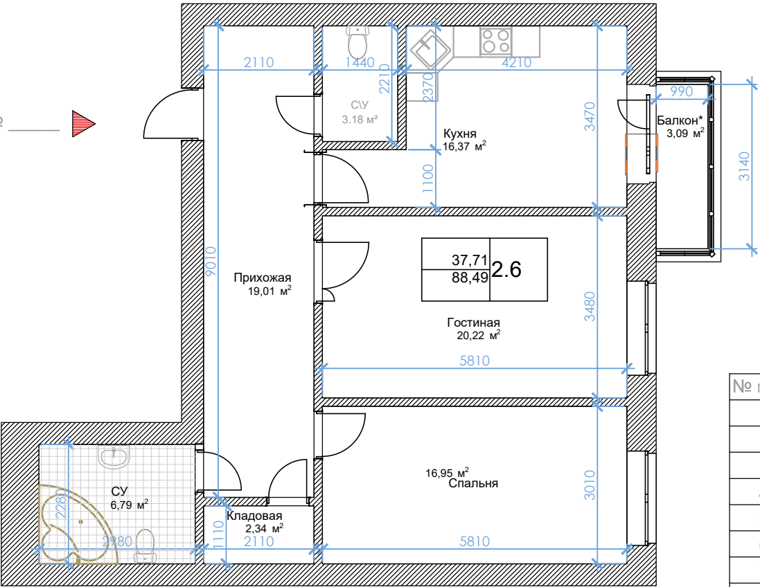
ЭКСПЛИКАЦИЯ ПОМЕЩЕНИЙ
