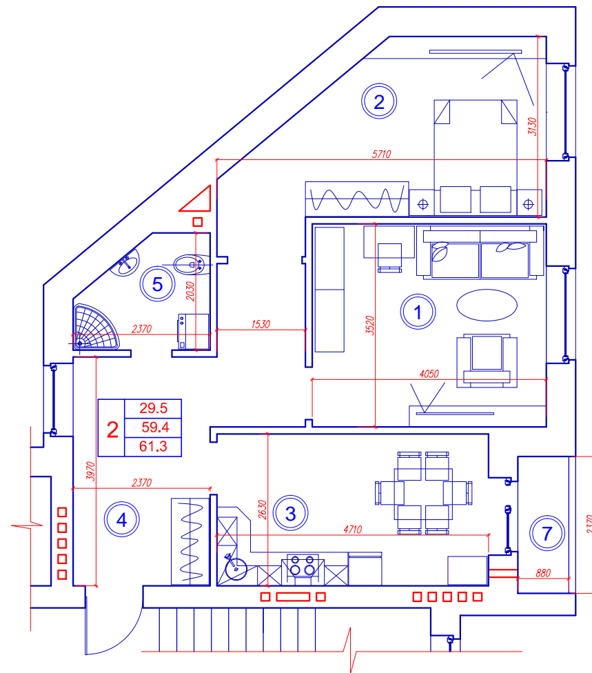
Двух комнатная квартира Блок -3. подъезд-7
