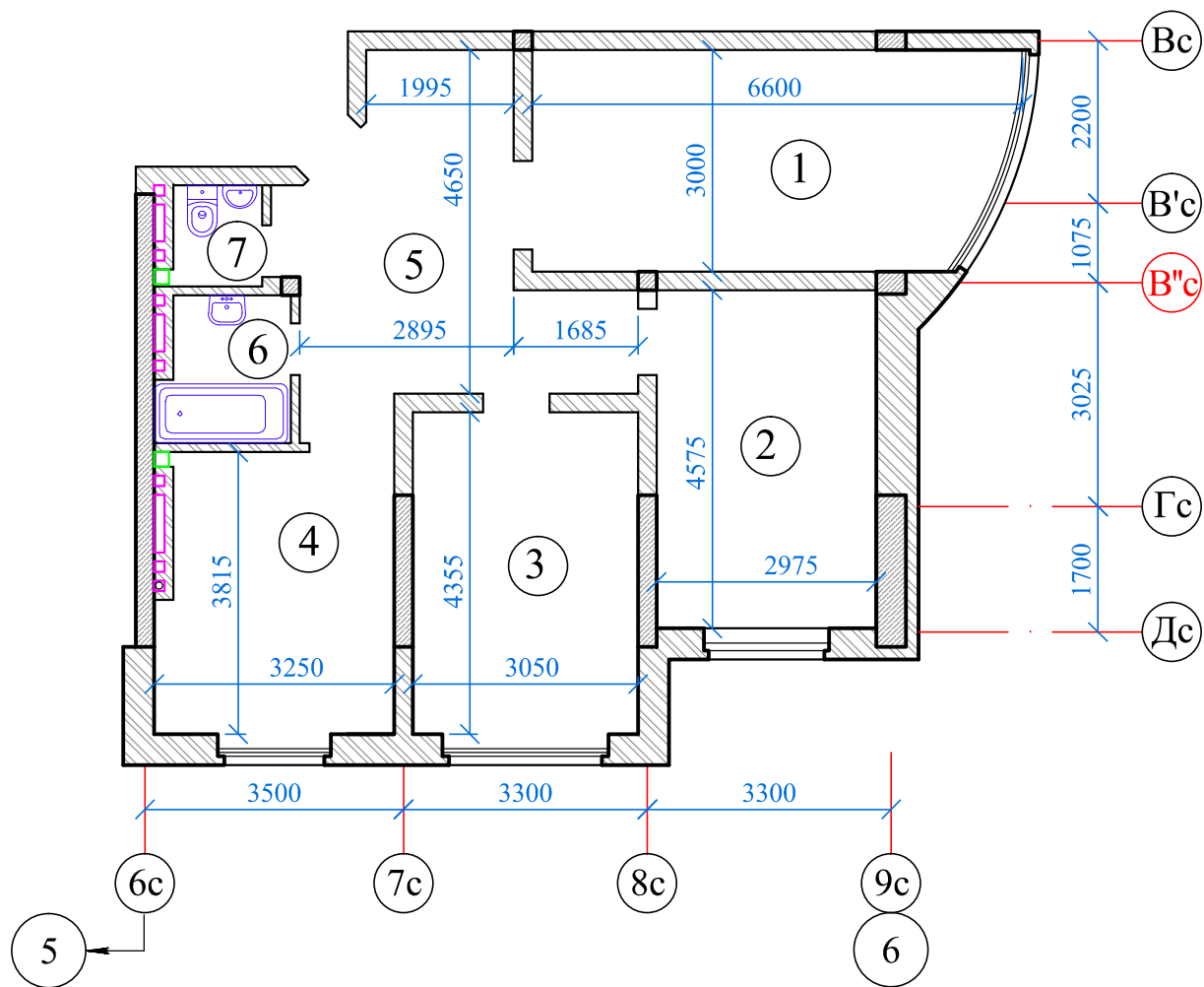
Экспликация помещений
